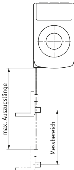
Abb. 1: Prüfung Auszugslänge
