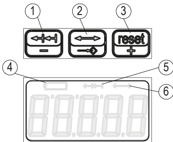
Abb. 3: Tastenfunktionen und Anzeigesymbole
